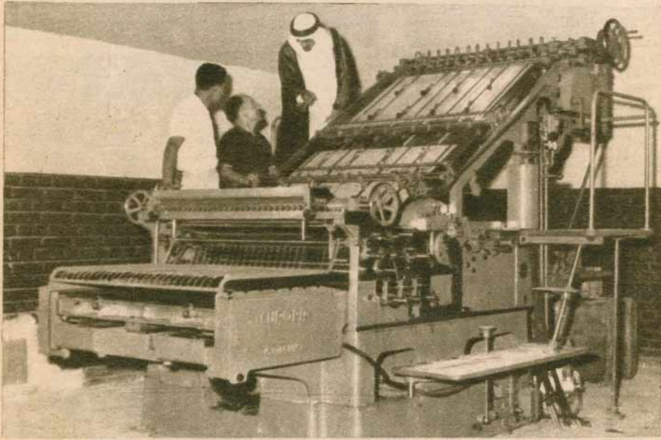
احدى ماكينات فرانكتال الكبيرة وهي تطبع في الساعة خمسة آلاف طبعة
